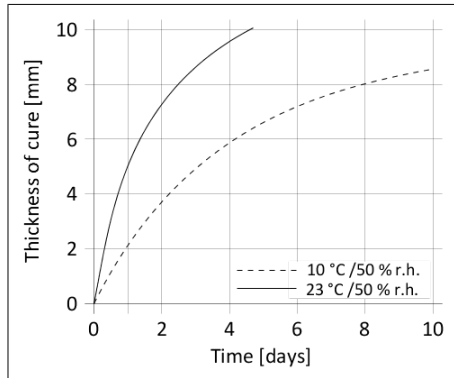
Diagrama 1: Velocidade de cura do SikaTack® Ultrafast
