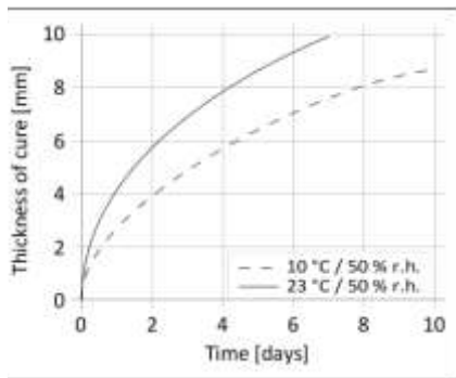
Diagrama 1: Velocidade de cura do Sikasil® Gasket Grey
