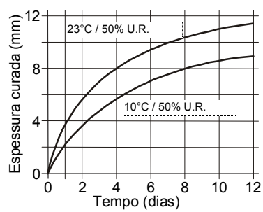
Diagrama: Velocidade cura Sikaflex®-227
