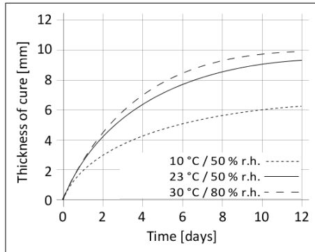
Diagrama 1: Velocidade de cura do Sikaflex®-558
