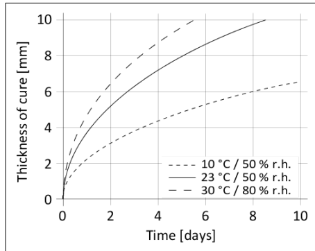
Diagrama 1: Velocidade de cura do Sikaflex®-254
